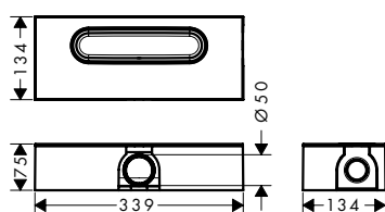
uBox universal za standardnu ugradnju
