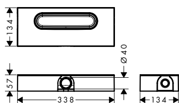
uBox universal za ravnu ugradnju
